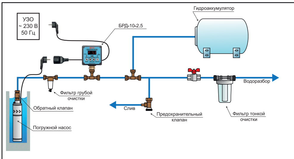
Пример 2. Подключение БРД к погружному насосу.
