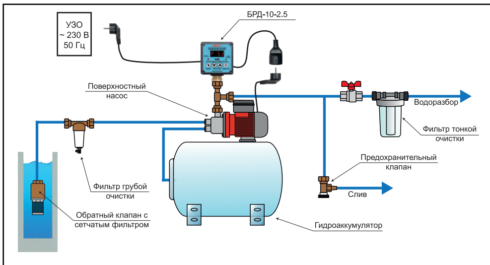
Пример 1. Подключение БРД к поверхностному насосу или насосной станции.
